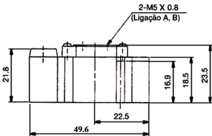
5/2 vias Simples Piloto - VYA3120
