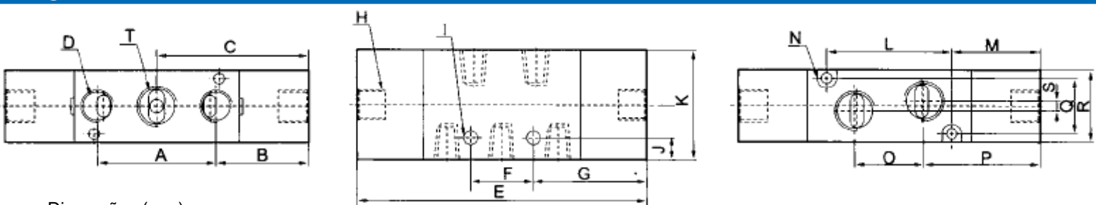
Dimensões (mm)
