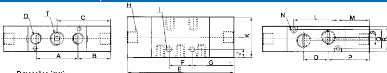
Dimensões (mm)
