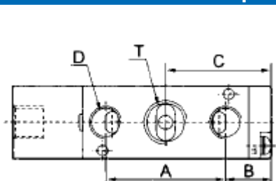
Dimensões (mm)
