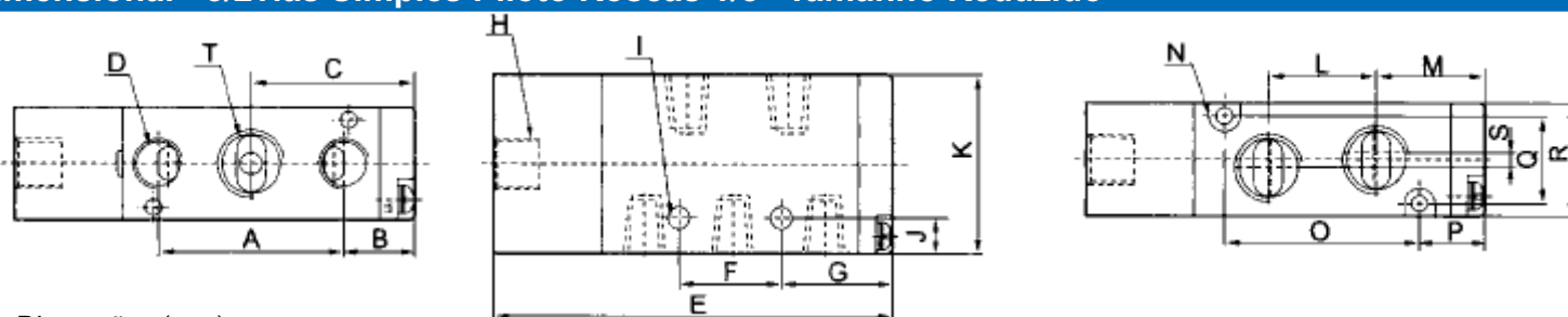
Dimensões (mm)
