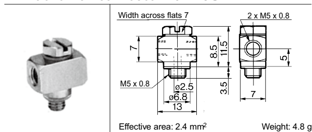
'T' Macho Fêmea Rosca M5: F-5UT
