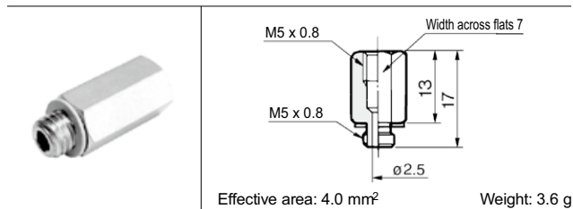
Extensor de R. Macho Fêmea Rosca M5: F-5J
