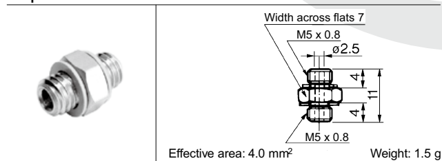
Nilpe Rosca M5: F-5N
